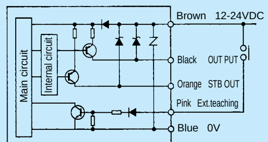
PNP output
