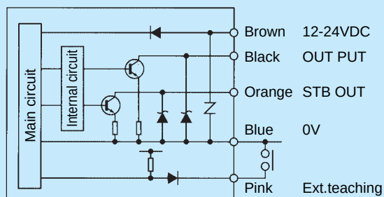
NPN output
